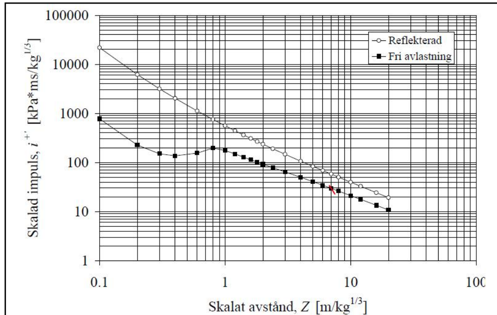
Figur 8. Reflekterad och oreflekterad impulsintensitet som funktion av det skalade avståndet Z (från SRV 2007).
