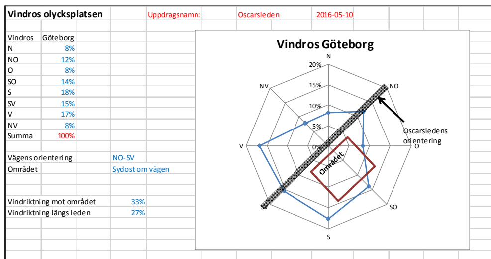
Figur 5b. Vindros för Oscarsleden
